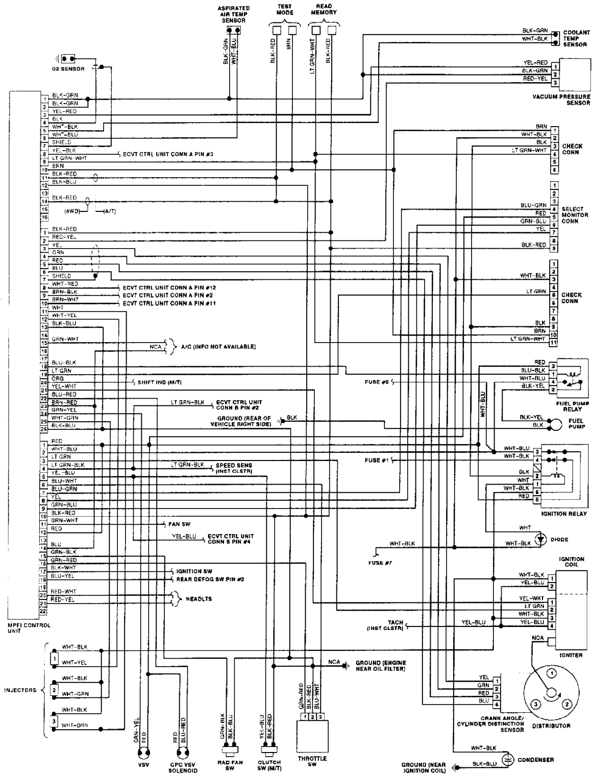
Fig. 2: Wiring Diagram (Justy 1.2L PFI)
